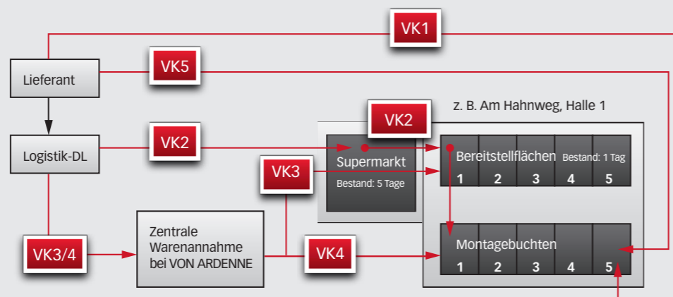
Abb. 6: Taktische Anlieferplanung nach Versorgungsklassen
